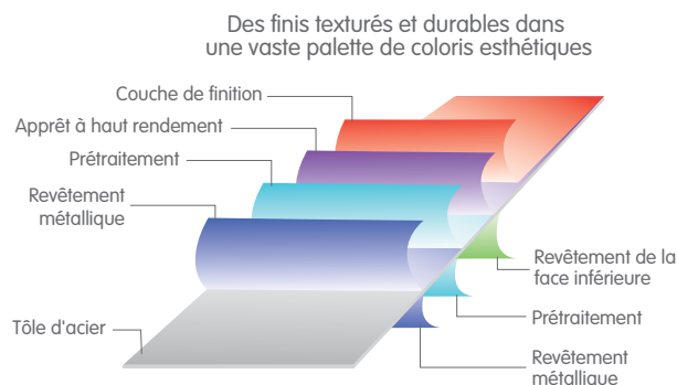
Figure 1: Caractéristiques du système de peinture
