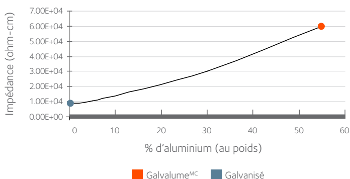
Impédance électrochimique de divers enduits d'alliage métallique aluminium-zinc
